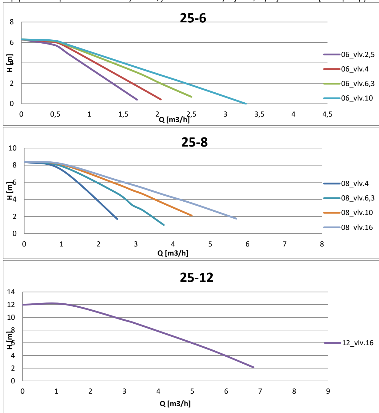
Rys.3. Charakterystyka pomp
