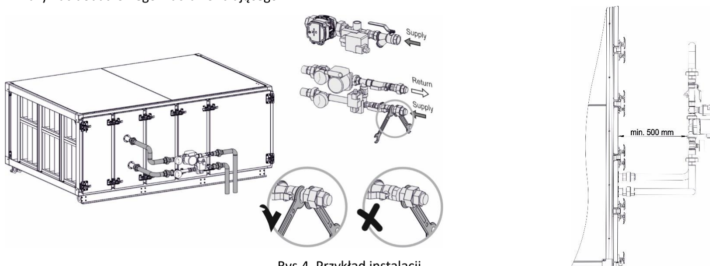
Rys.4. Przykład instalacji
